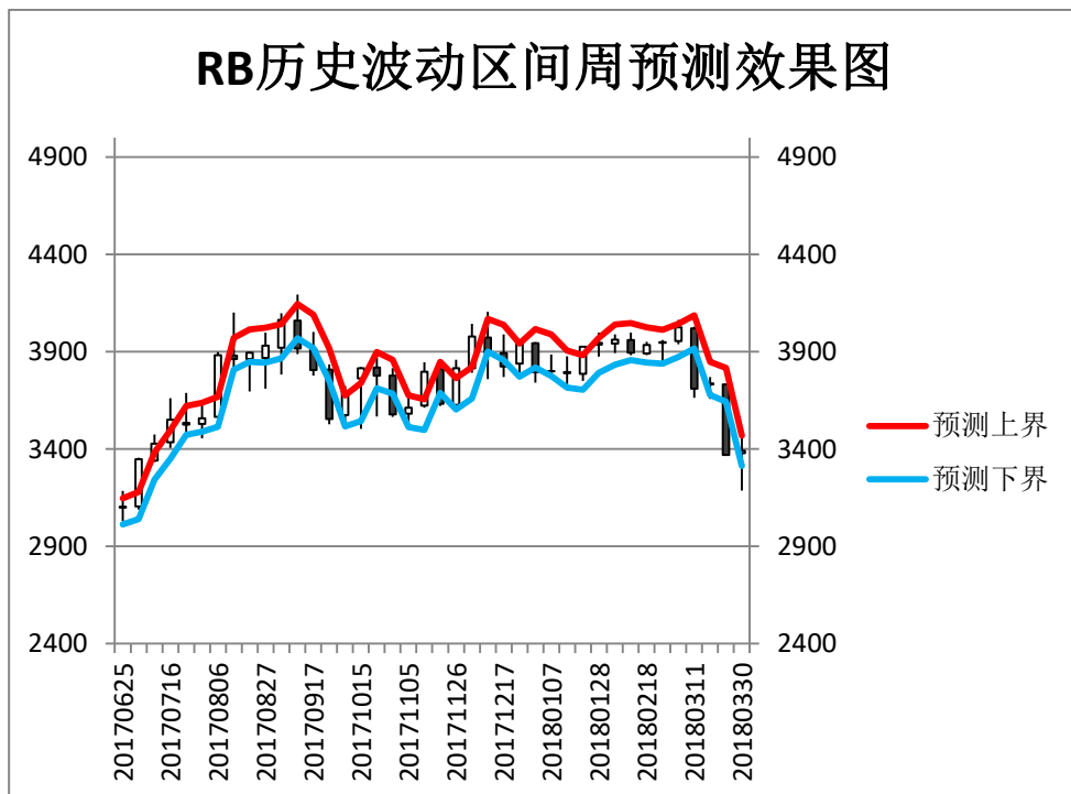
RB 历史波动区间周预测效果图
