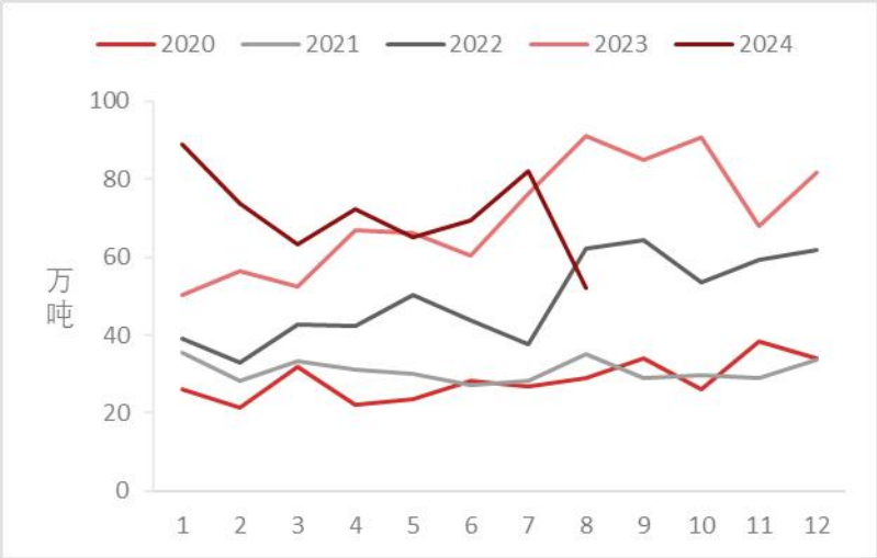
镍铁进口量
