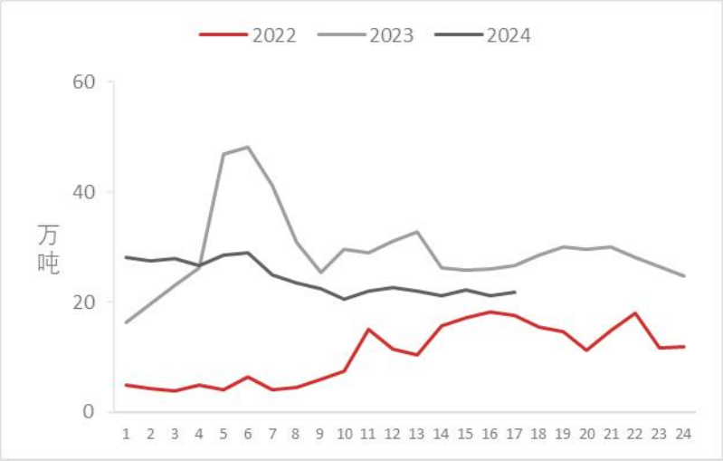
镍铁库存
