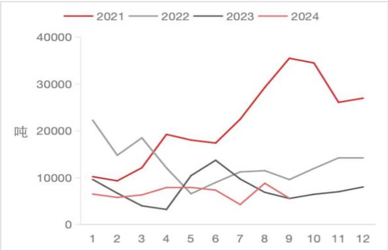
纯镍出口量
