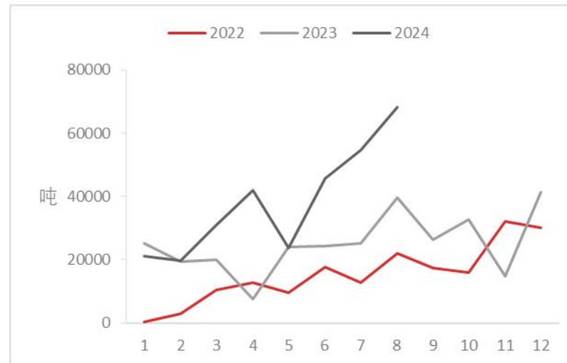
镍铈进口量
