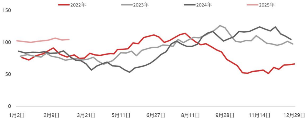
MTO/MTP 开工率
