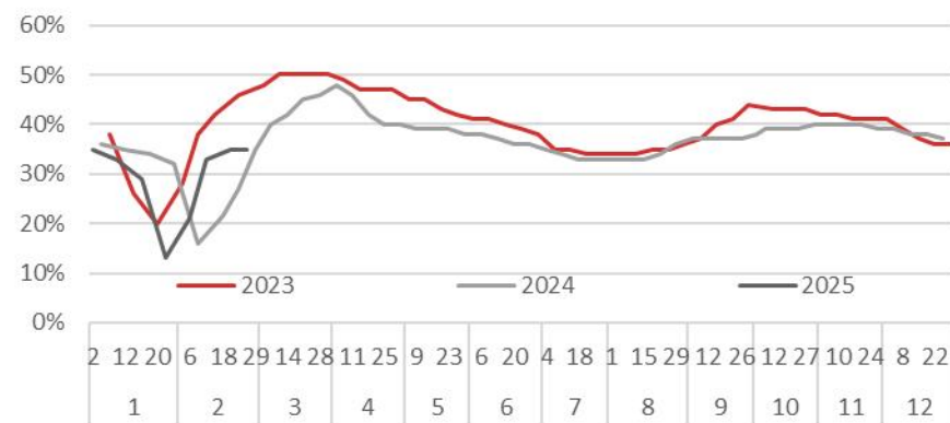
管材开工率
