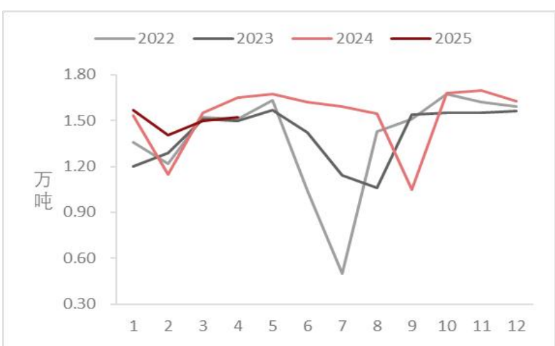
精炼锡产量
