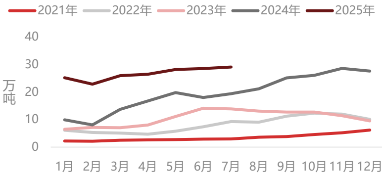
磷酸铁锂产量（月）
